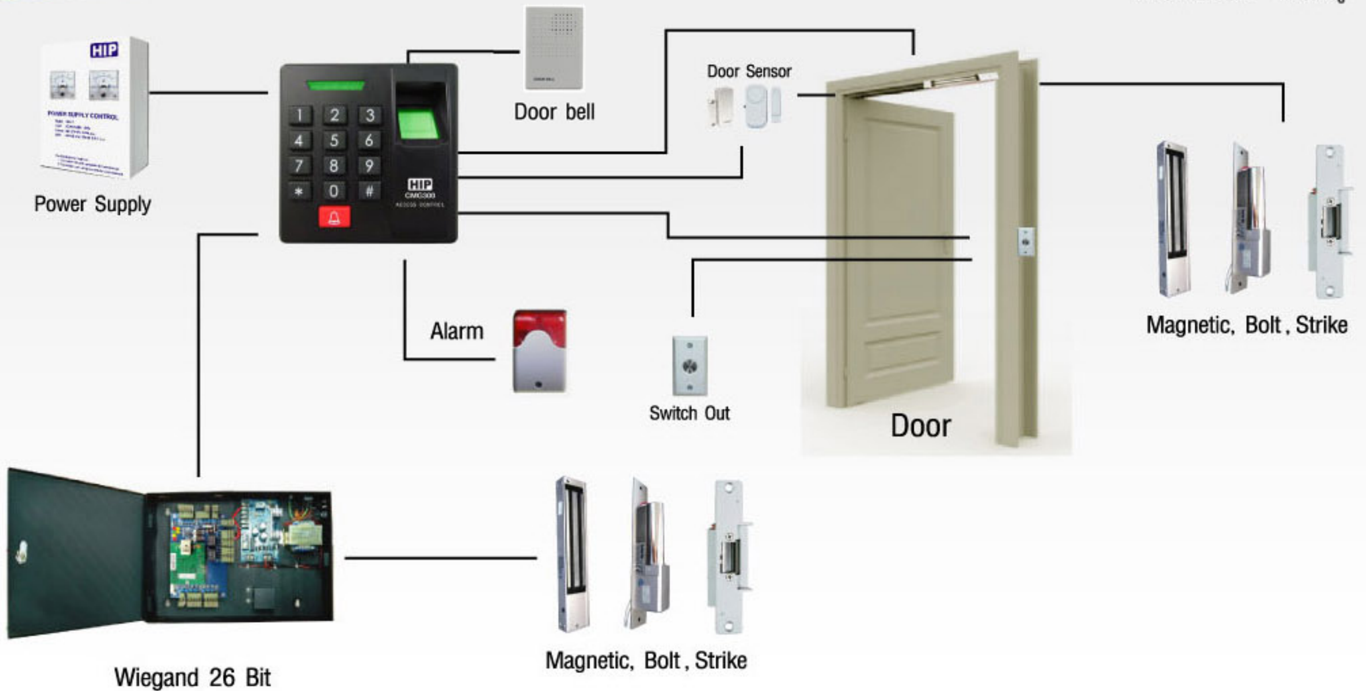
Installation Diagram Standalone การทำงานเปิด - ปิดประตู
